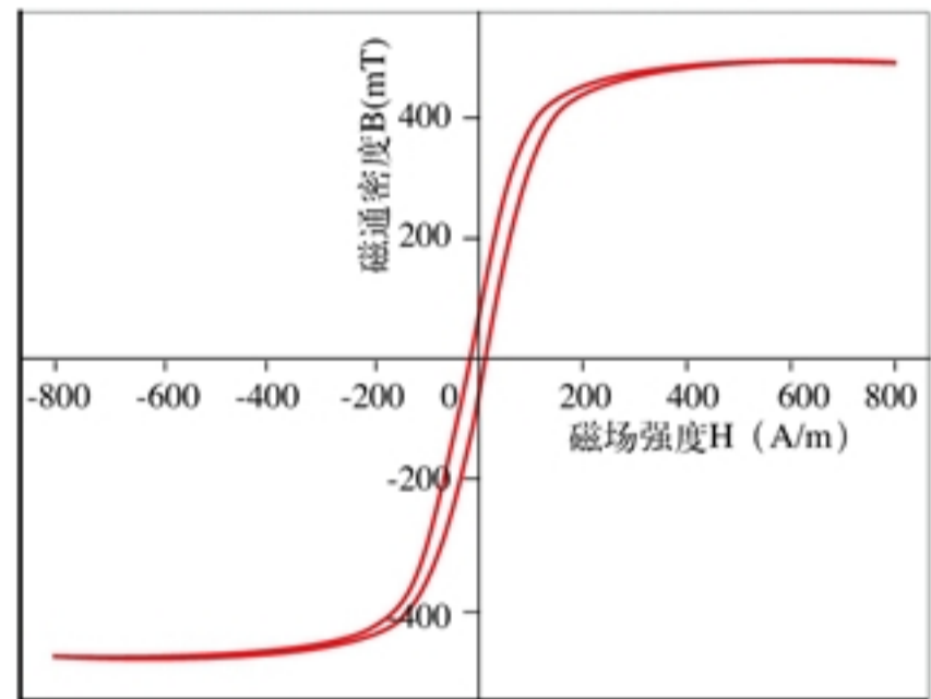
R2KB&R2KB1 磁滞回线(B-H)
