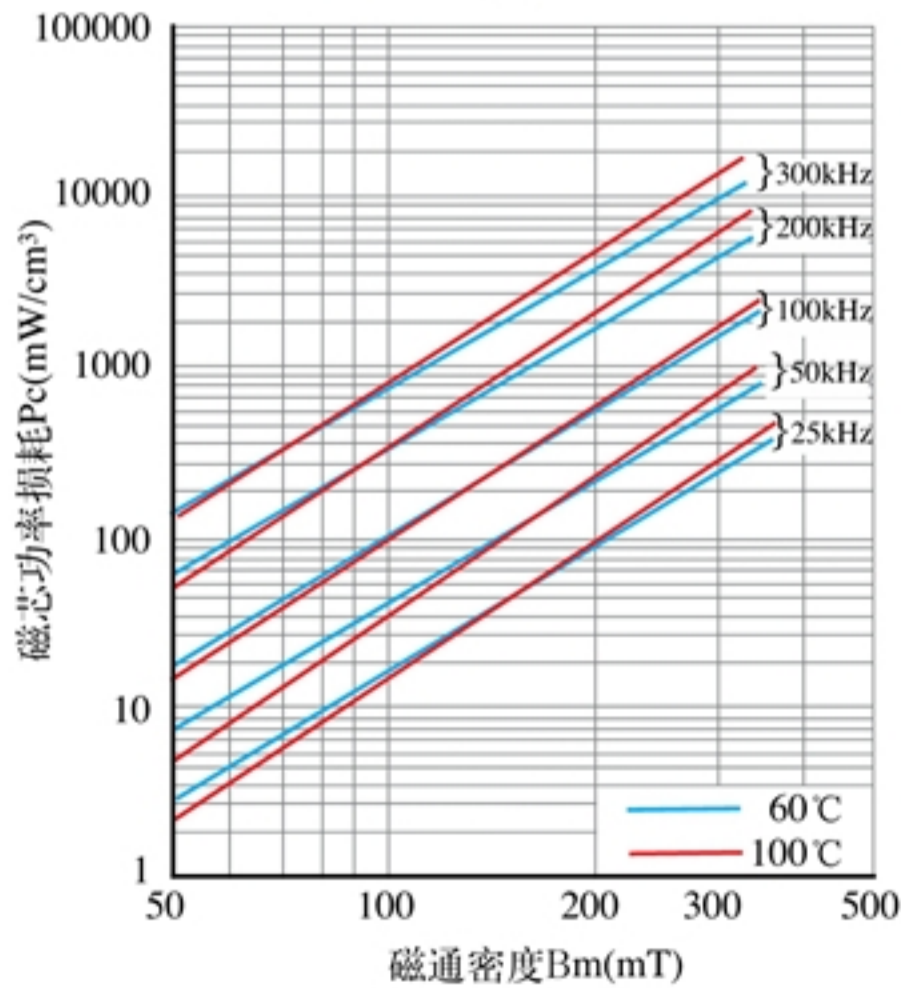
R2KB 功耗曲线
