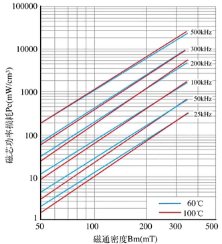
R2KB1 功耗曲线
