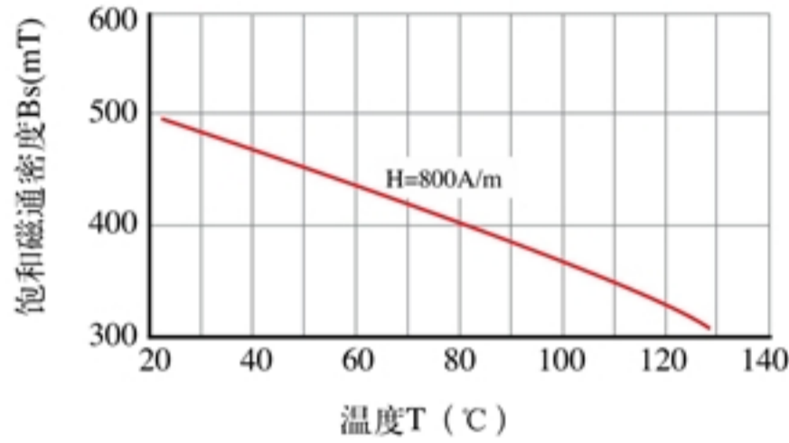
R2KB&R2KB1 饱和磁通密度随温度变化(Bs-T)
